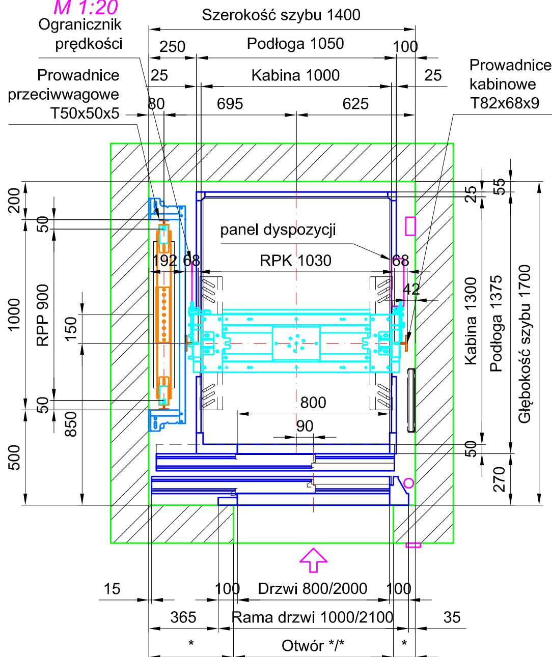
PRZEKRÓJ PRZEZ SZYB Rama kabinowa: TLM9/TLM10 M 1:20
