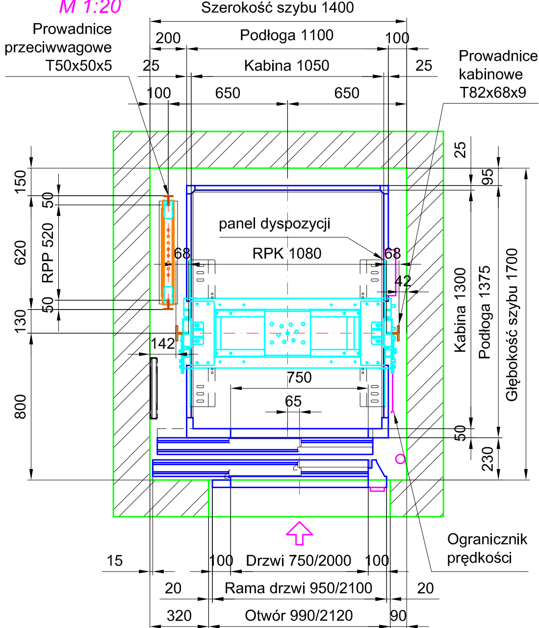
PRZEKRÓJ PRZEZ SZYB Rama kabinowa: TLM9/TLM10 M 1:20
