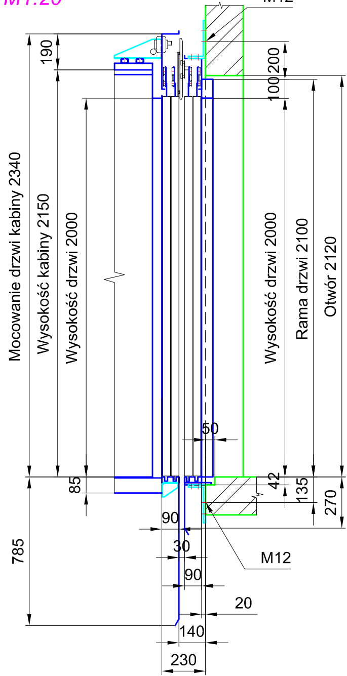
DRZWI PRZYSTANKOWE KABINOWE KLEFER 2P (MODEL 40/10 PM) M1:20
