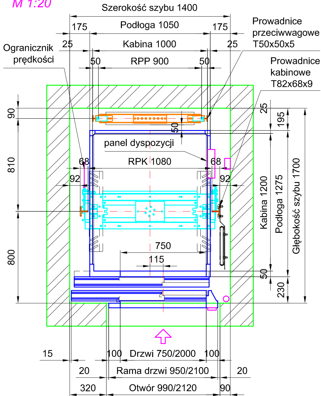
PRZEKRÓJ PRZEZ SZYB Rama kabinowa: TLM9/TLM10 M 1:20
